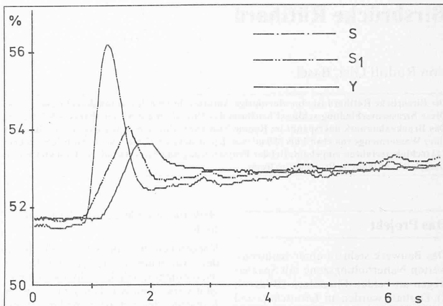
Bild 11. Anfangsbereich der Übergangsfunktionen der PID-Regleinrichtung einer Pumpturbine des Pumpspeicherwerkes Kühltai der Tiroler Wasserkraftwerke AG.
