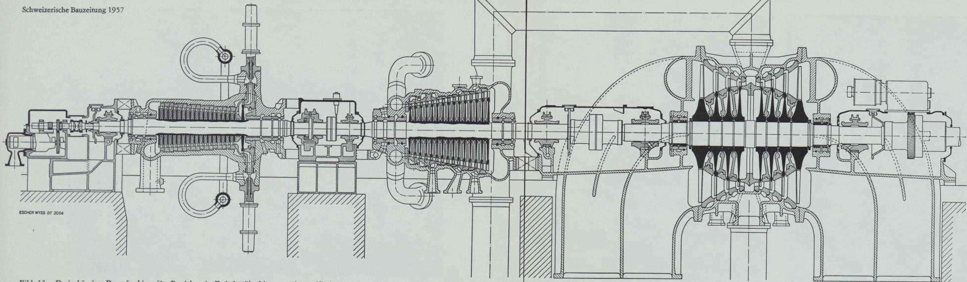
Bild 13. Dreigehäusige Dampfturbine für Betrieb mit Zwischenüberhitzung mit zweiflutigem Niederdruckteil; Leistungsklasse 60 bis 80 MW für kaltes Kühlwasser oder 100 bis 120 MW für rückgeköhltes Kühlwasser
