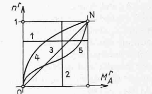
Bild 24. Drehzahl-Drehmoment-Kennlinien der Arbeitsmaschine in relativen Grössen:
