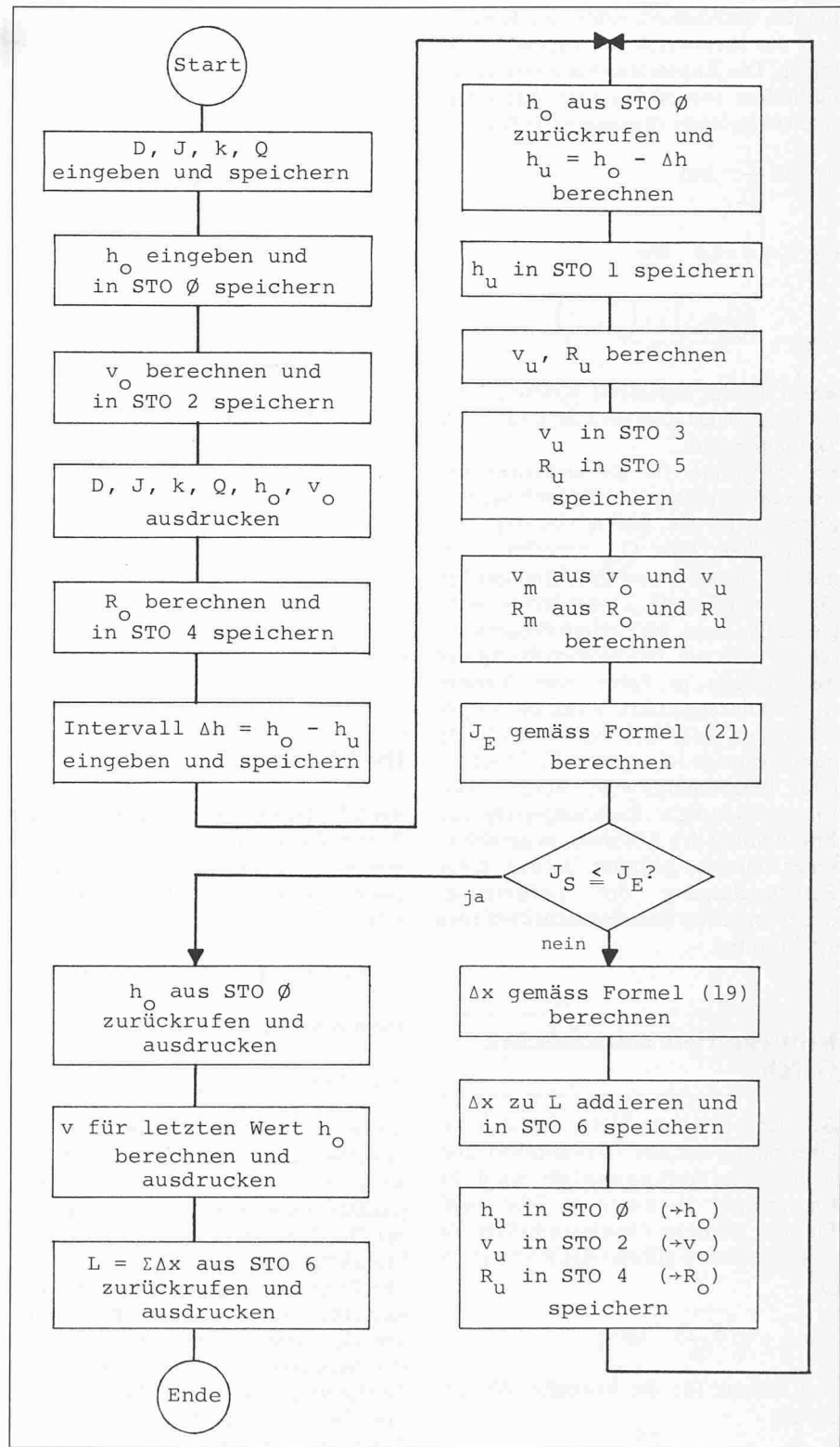
Bild 4. Strukturdiagramm für die Berechnung der Senkungslinie gemäss Formeln (19) und (21). L = \sum \Delta x stellt die Summe der einzelnen um Intervall \Delta h = h_0 - h_u differenzierten Querschnittsabstände der Rohrleitung dar
