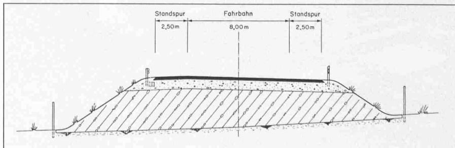
Normalprofil Autostrasse
