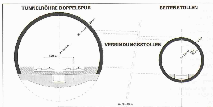
Bild 2. Vorgesehenes Lichtraumprofil
