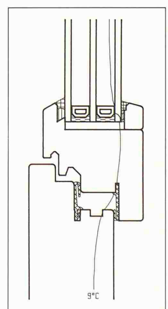
Bild 6. Detail A4, entspricht in Konstruktion dem Detail A2, jedoch Isolierglas-Randverbund mit Distanzstege in Kunststoff statt Stahl
