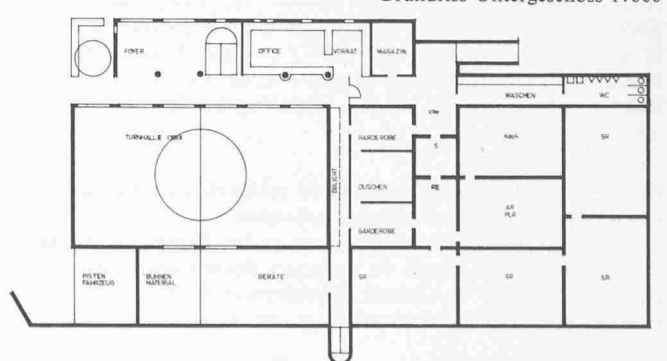
Grundriss Untergeschoss 1:800
