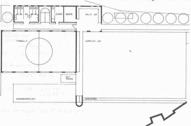
Grundriss Erdgeschoss 1:800
