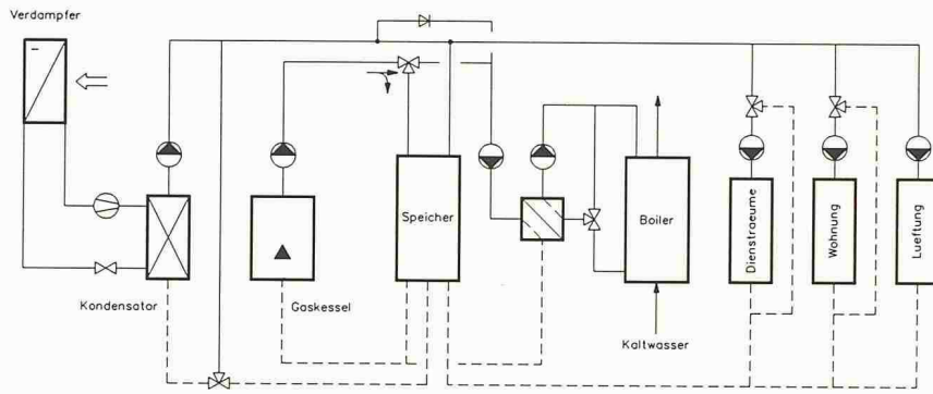
Prinzipische der Anlage: Elektrowärmepumpe mit Luft und teilweiser Abwärme als Wärmequelle, bivalent alternativ (-3 °C), Heizleistung 43.2 kW (50/45 °C, -1.5/-7.3 °C), Leistungsziffer 2.8
