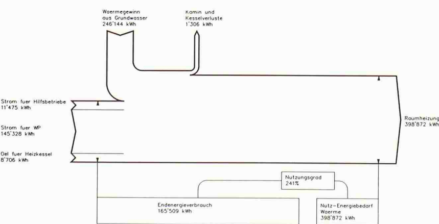
Energie-Flussdiagramm 1984-1985
