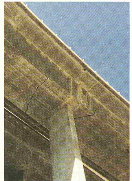
Bild 5. Reussbrücke Wassen, Aufreissen des Überbaus durch Absenken der Fundation Bildautor: R. Kalbermatten
