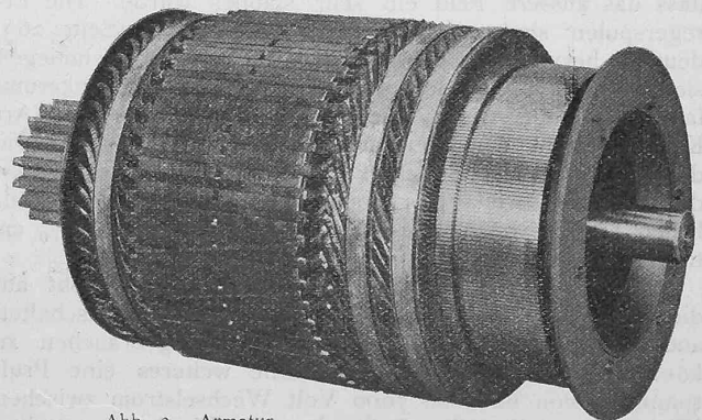
Abb. 3. Armatur.
