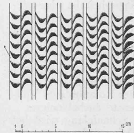
Schaufelung im Schnitt a - b.
