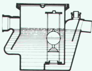
PASSAVANT-Klein-Benzinabscheider
