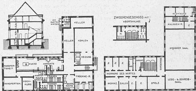
Typus B, Gemeindehaus. I. Preis, Entwurf Nr. 49. — Verfasser: H. Vogelsanger und A. Maurer, Architekten in Rüslikon.
