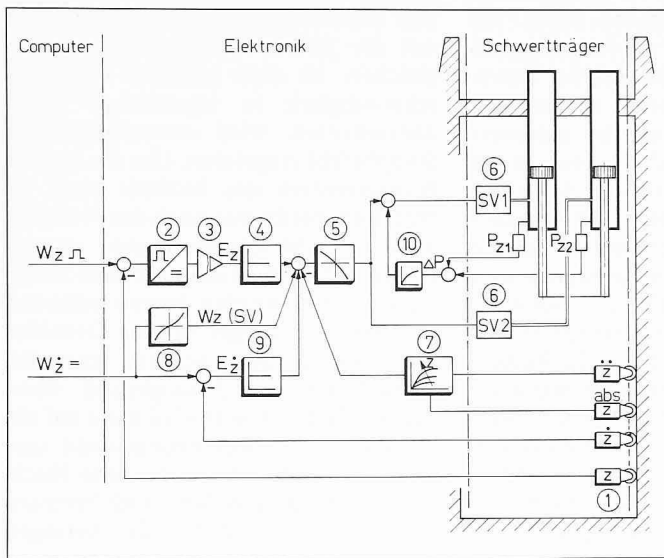
Bild 7. «Normal Use»-Regelungssystem
