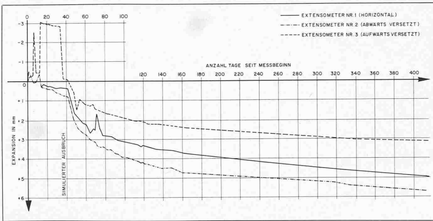
Bild 5. Ergebnisse der Langzeit-Deformationsmessungen in der Versuchskaverne. Messungen im Auftrag der ARGE Huttegg, ausgeführt von der Terrexpert AG, Bern
