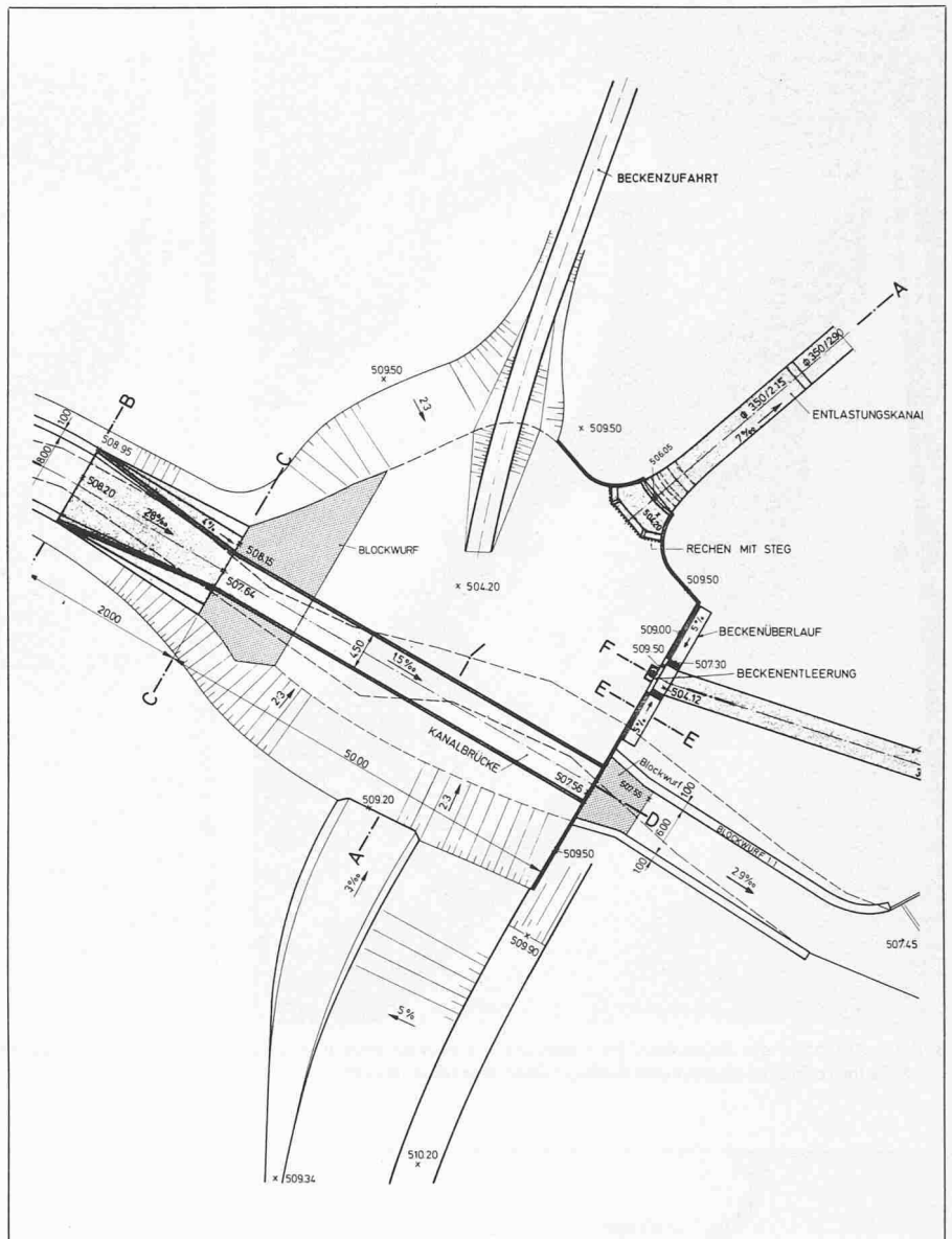
Bild 6. Verzweigungsbauwerk mit Brücke. Das Wasser der Langeten wird über eine Brücke geführt, die über einem Becken angeordnet ist. Bei einem Abfluss von 12 m³/s erreicht der Wasserspiegel die Überlaufkanten. Bei zunehmendem Hochwasser fällt das Überschusswasser Q 2 in ein Sammelbecken und wird von dort aus in einen überdeckten Kanal geleitet
