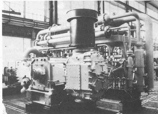
Fünfstufiger Burckhardt-Boxer-Kompressor (2700 m 3 Luft/h, 139 bar abs, 580 kW) liefert die Druckluft für die Luftkanonen
