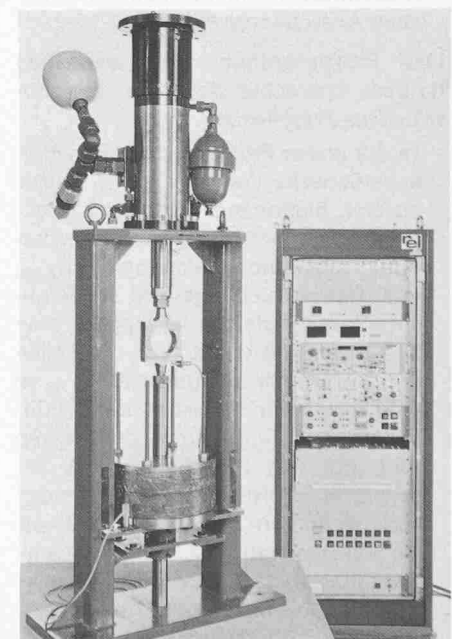
Bild 4. Servohydraulischer Schwingungserreger
