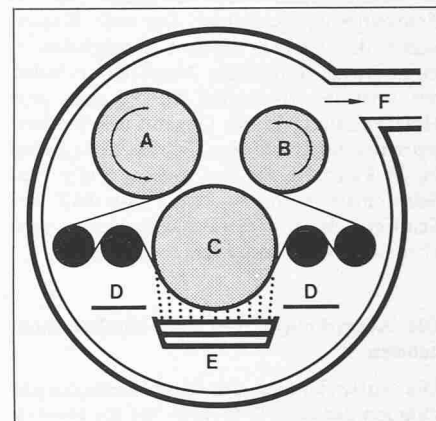
Schema einer Metallisierungsanlage: A: Aufwickelrolle, B: Abwickelrolle, C: Kühltrommel, D: Hitzeschild, E: Metallquelle, F: Pumpe. Durch dieses Verfahren gewinnt die Polyesterfolie Metallcharakter, Licht-, Wärmereflexion und eine verbesserte Gassperre
