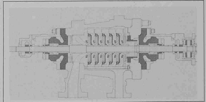
Schnitt einer mehrstufigen Sulzer Mantelgehäusepumpe Typ GSG
