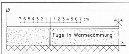
Bild 3. Modell für die Berechnung mit der Methode der finiten Elemente. Annahmen: ebener Verformungszustand, Wand als Untergrund starr, Verputzaufbau homogen und einschichtig
