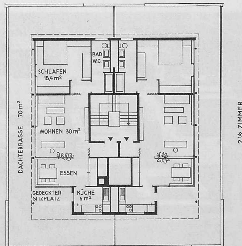
Attikageschoss der Turmbauten, 1:300
