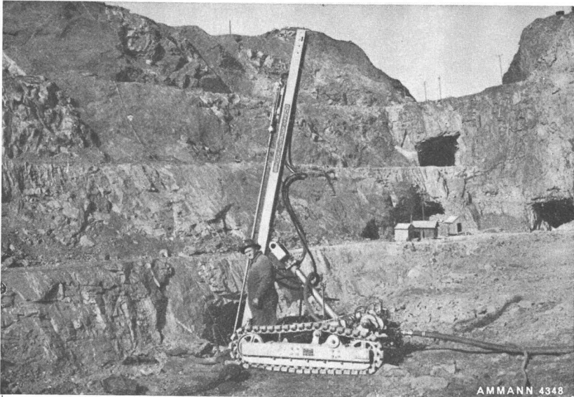
AMMANN 4348
