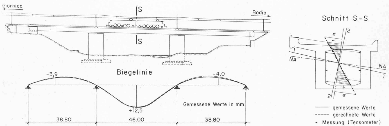
Bild 6. Belastungsprobe. Biegelinie und Spannungen in Systemmitte bei Belastung mit einer Lokomotive Ae 8/14 (246 t) in Mittelfeld. E_b = 420 \text{ t/cm}^2
