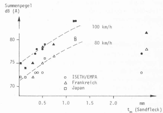
Bild 12. Summenpegel der Rollgeräuschkartenentwicklung in Funktion der mittleren Texturtiefe
