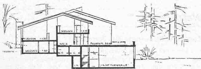
Schnitt Lehrerzimmer-Turnhalle 1:600
