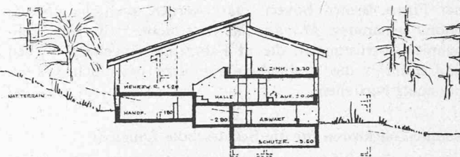
Schnitt Mehrzweckraum-Abwart 1:600
