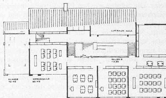
Grundriss Galeriegeschoss 1:600
