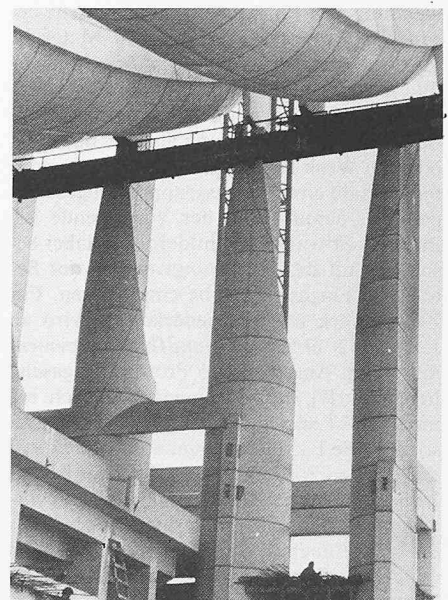
Bild 8. Regierungsbäude in Kuwait aus Stahlbetonfertigteilen nach niederländischen Entwürfen und Herstellungsverfahren
