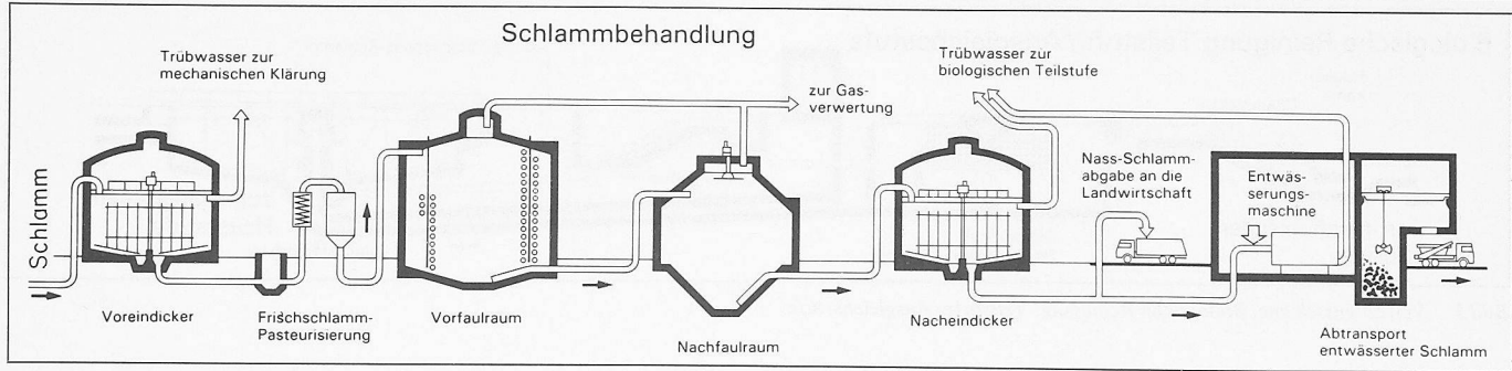
Bild 7. Verfahrensschema, Schlammbehandlung
