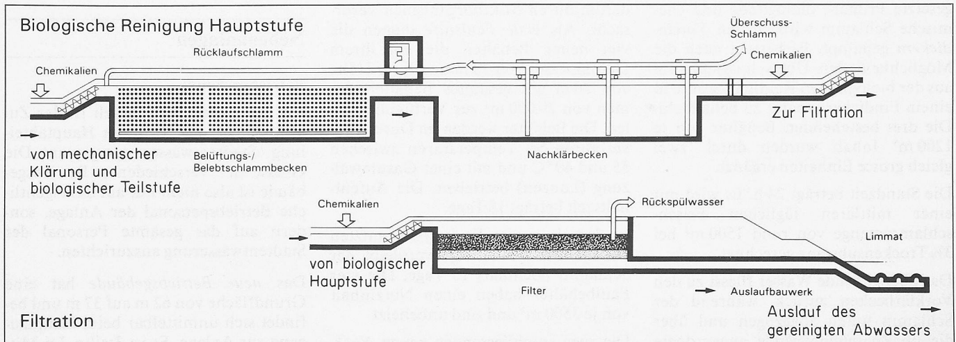
Bild 6. Verfahrensschema. Biologische Reinigung Hauptstufe (oben) und Filtration (unten)
