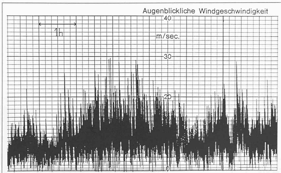
Bild 5a. Windgeschwindigkeitsaufzeichnung
