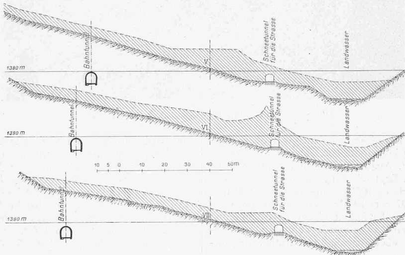
Abb. 5. Querprofile zu Abb. 4. Rutschobel- und Stützbug-Lawine, März 1907. — 1 : 1500.
