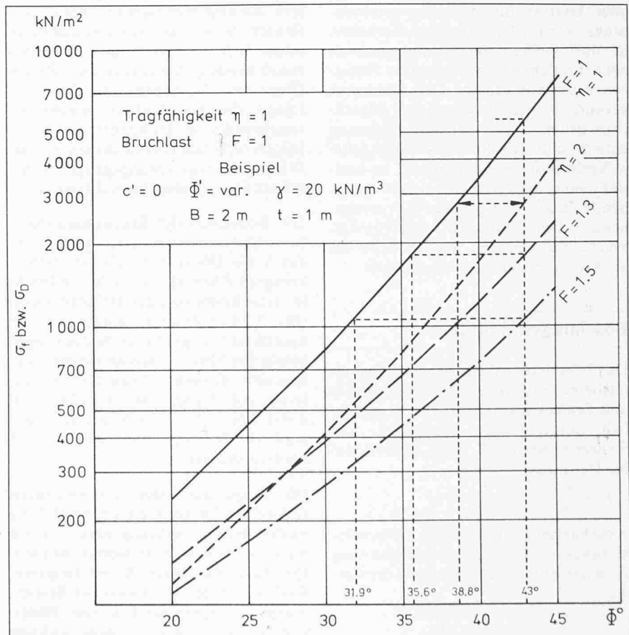
Bild 4. Beispiel zur Tragfähigkeit eines Streifenfundamentes: Auswirkung der unterschiedlichen Definition von \eta und F in Abhängigkeit vom Reibungswinkel \Phi
