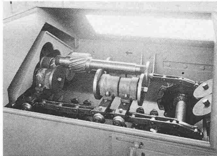
Bild 19. Blick in die Beladestation einer Durchlaufmaschine für das Peenen von Getriebewellen, Stirnrädern usw. mit Transportsystem für die Werkstücke gemäss Schema Bild 18A. Unmittelbar vor dem Eintritt in Strahlraum (links im Bild) ist eine auf den Drehvorrichtungen der Traversen liegende Getriebewelle zu sehen. Photo: Graber und Wening AG., Neftenbach
