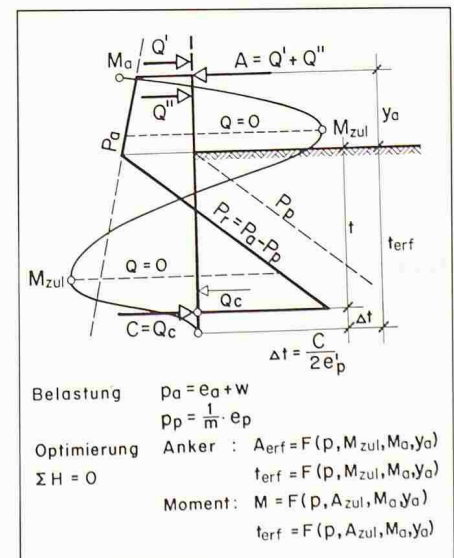
Bild 4. Berechnungsmodell Wandstatik; Bemessungsfall Wandfuss eingespannt
