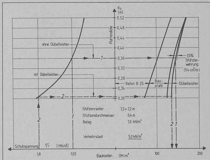
Bild 1. Linienzug 1-1. Plattendicke und zugehörige Baukosten, bei der ausser dem hohen Bewehrungsgrad von μg=1,5% gerade noch keine besonderen Massnahmen für die Sicherheit gegen Durchstanz erforderlich sind, wobei τ zul = 1,3 · 1,3 · √1,5 · 0,5 [MN/m 2 ]
