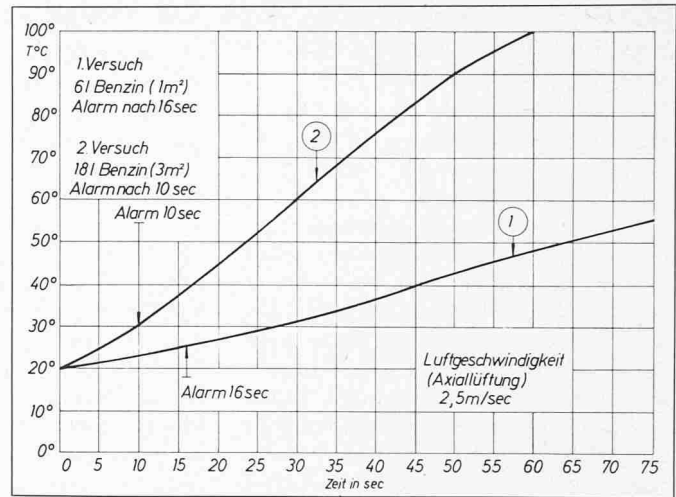
Bild 2. Abruggtunnel Zürich: Temperaturverlauf und Alarmauslösung in Funktion der Zeit
