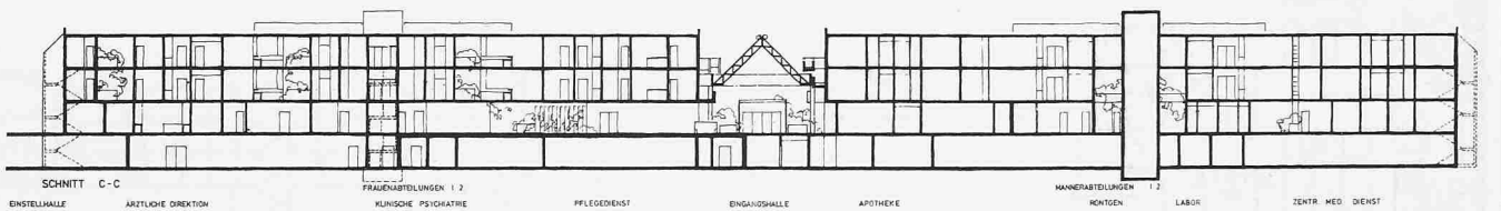
Schnitt C-C 1:800
