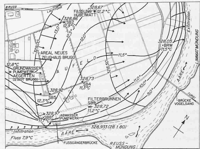
Bild 8. Temperaturverlauf [°C] und Isohyphen des Grundwasserspiegels (28.1.80)
