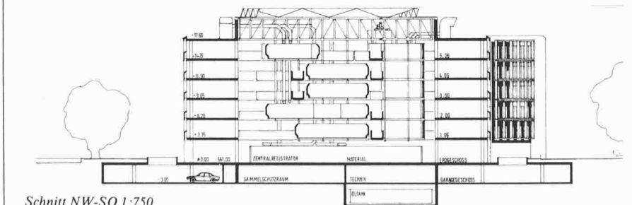
Schnitt NW-SO 1:750
