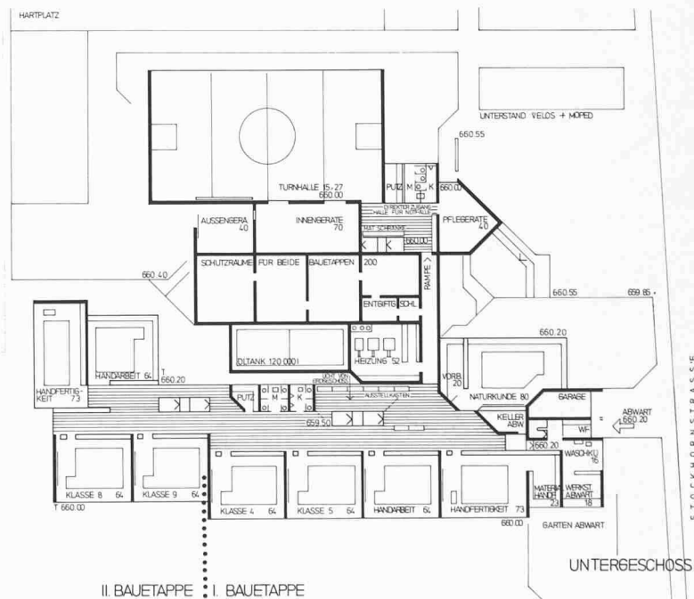
Grundriss Untergeschoss 1:800
