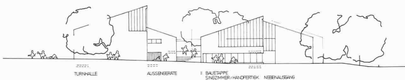
Schnitt Turnhalle-Eingangshof-Schultrakt 1:800
