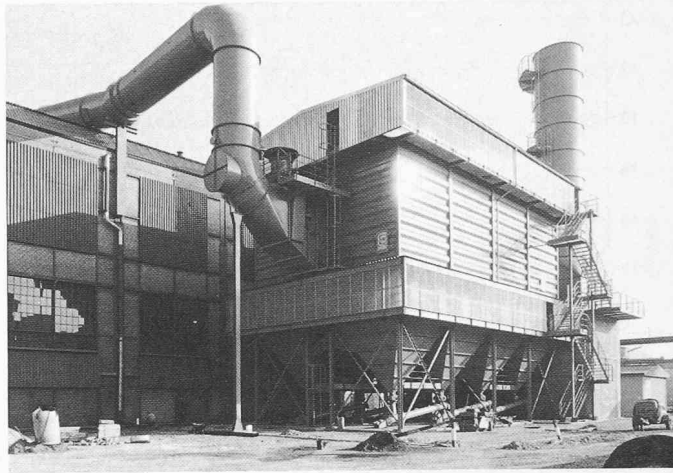
Bild 2. Der in der Einhausung erfasste Staub wird in ein Filterhaus abgesaugt, im Staubbunker gesammelt und als Granulat einem Recyclingverfahren zugeführt
