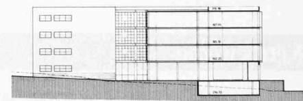
Sezione B-B
