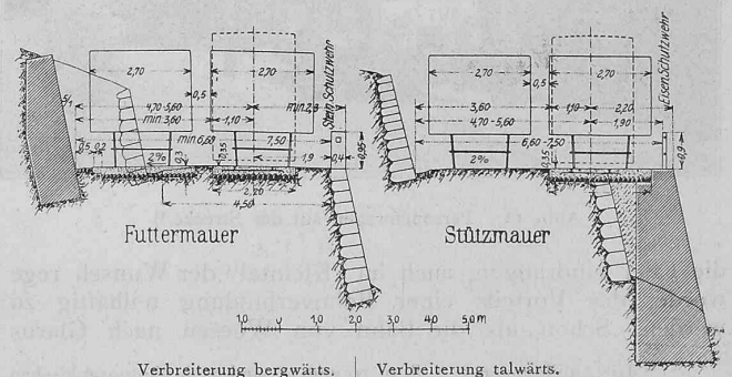
Abb. 3. Strassenprofile mit Verbreiterung. — Masstab 1 : 200.
