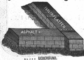
ABDECKUNG VON FUNDAMENTEN.
