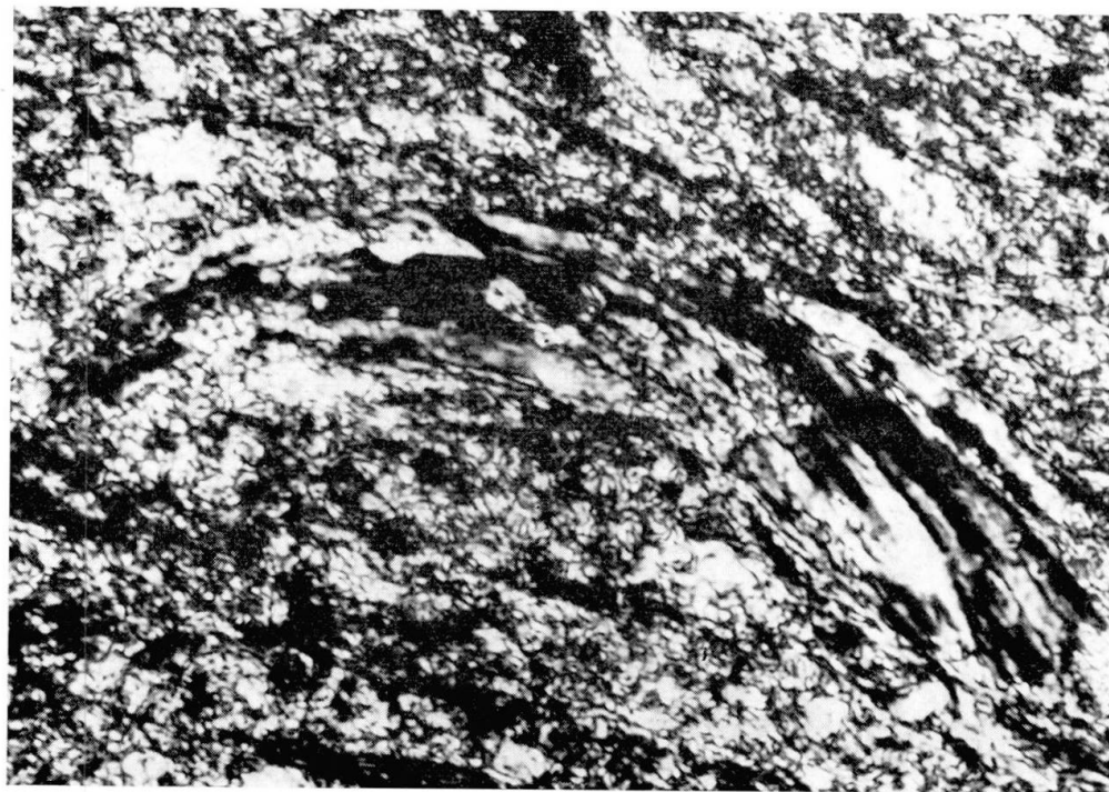
Fig. 9. Albit, deformiert an 2. Schieferung, Detail aus Fig. 8. Bildbreite 600 \mu .
