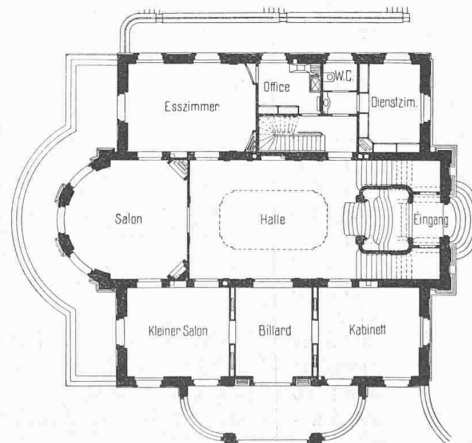
Abb. 3. Grundriss vom Erdgeschoss. — 1 : 400.
