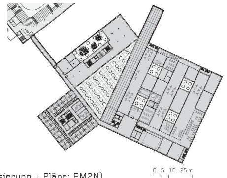
03+04 Grundrisse EG, 2. OG, Mst. 1:1500 (Visualisierung + Pläne: EM2N)
