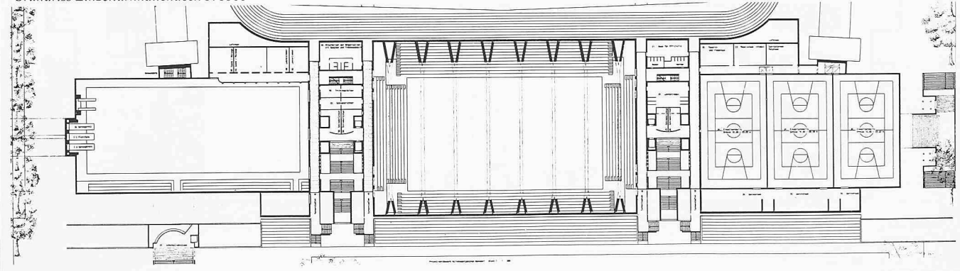
Grundriss Einzelturnhallendeck 1: 1300
