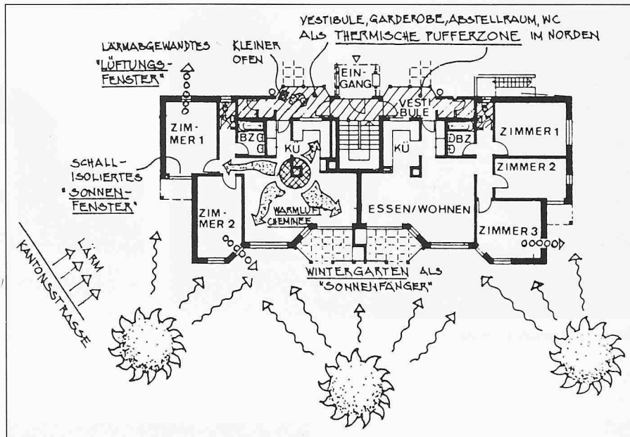
Bild 6. Grundriss
