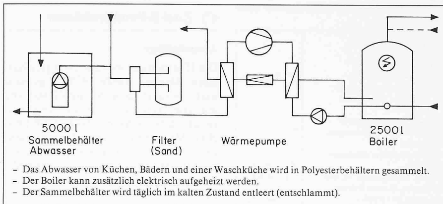
Bild 15. System-Beschrieb für die Warmwasseraufbereitung
