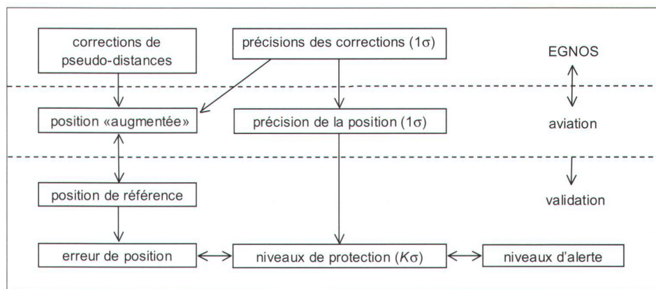
Fig. 3: Le concept d'intégrité d'EGNOS.
